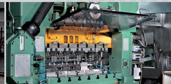
Modulares Folgeverbundwerkzeug
